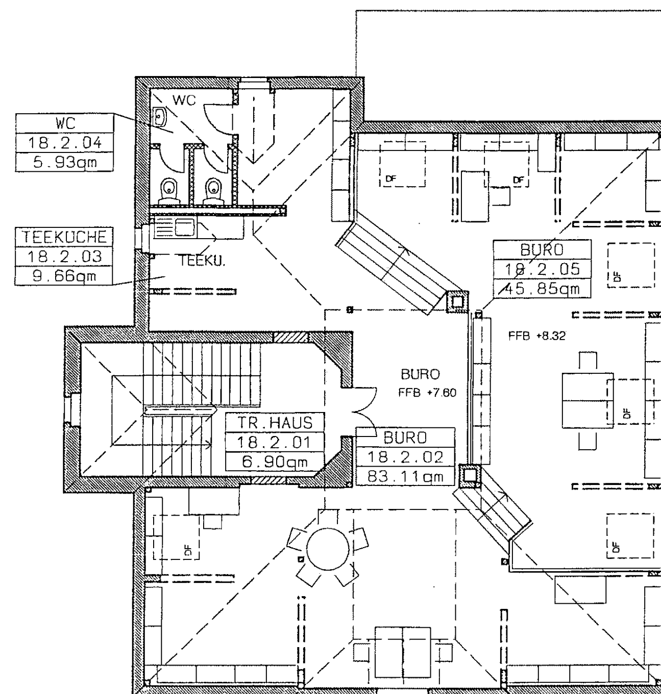
GRUNDRISS DACHGESCHOSS
