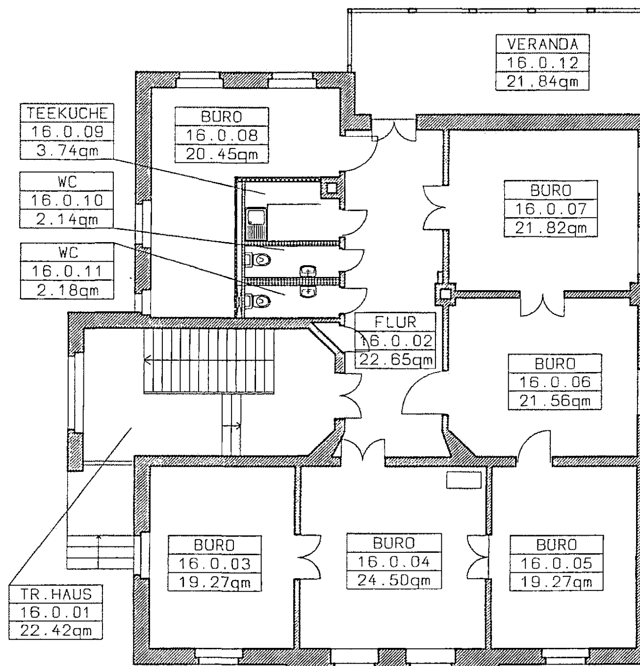
GRUNDRISS ERDGESCHOSS
