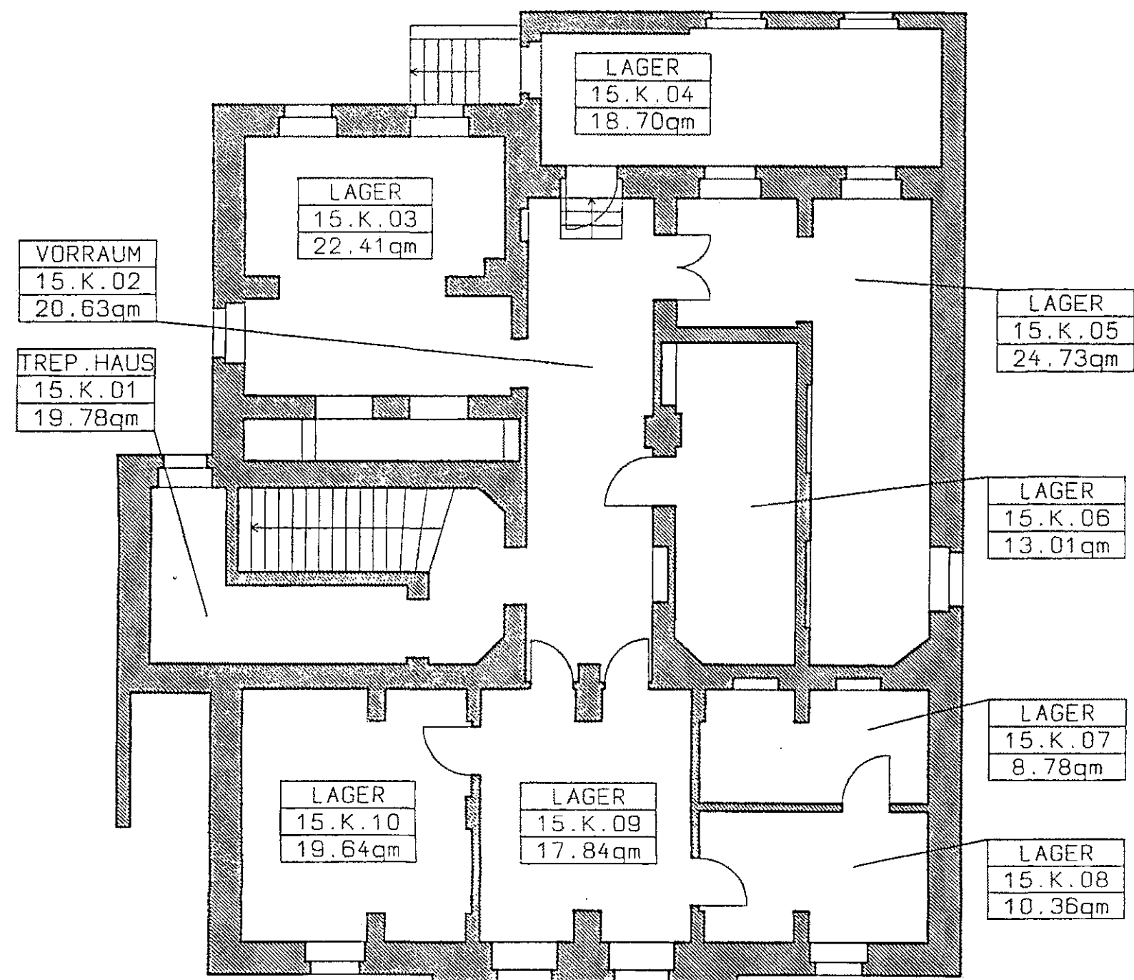
GRUNDRISS KELLERGESCHOSS
